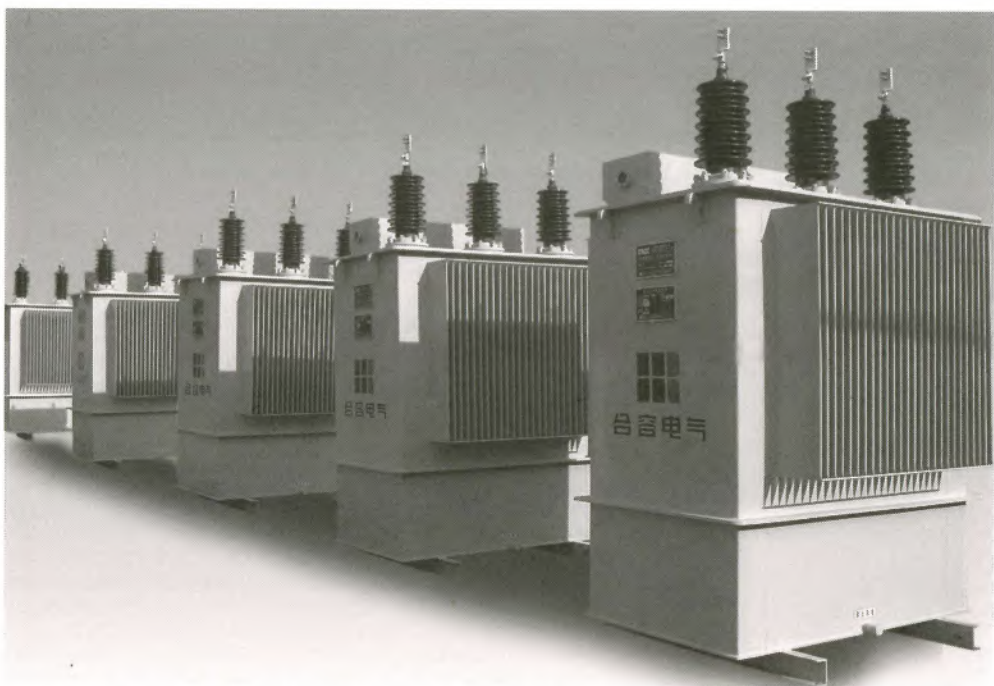
合阳电力电容器制造有限公司生产的高科技产品 35kV 集合式并联电容器
